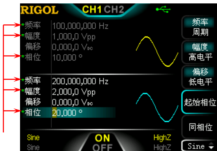
图 2-20 通道耦合
