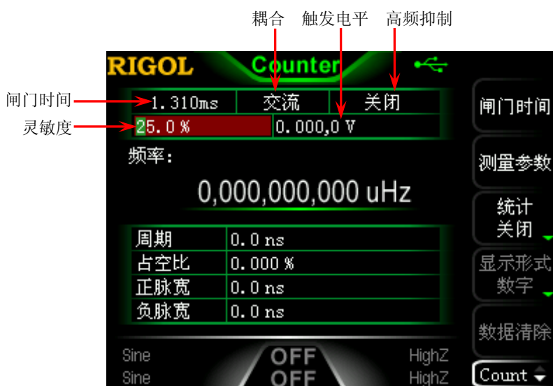
图 2-13 频率计参数设置界面
