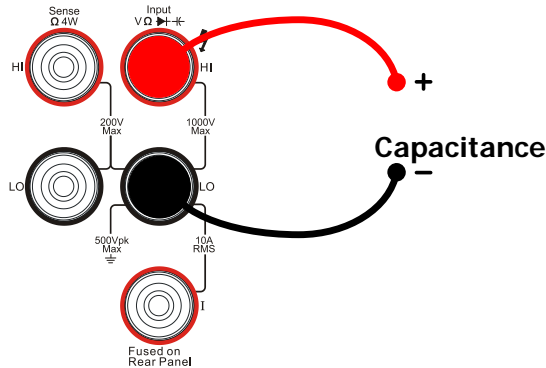
图 2-24 电容测量连接示意图
