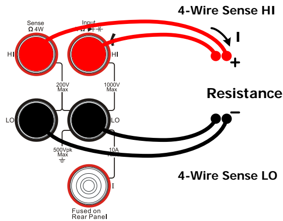
图 2-21 四线电阻测量示意图
