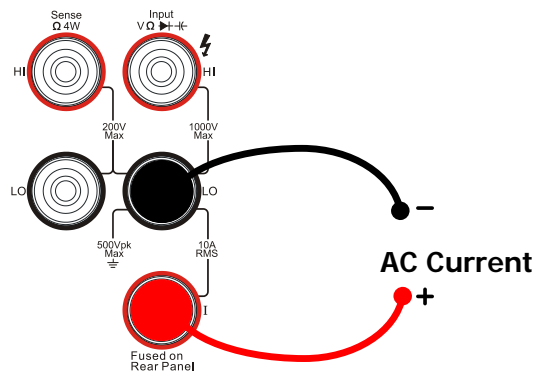
图 2-15 交流电流测量连接示意图
