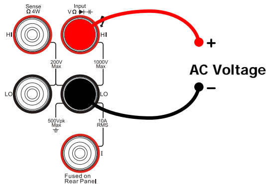
图 2-8 交流电压测量连接示意图
