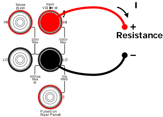
图 2-18 二线电阻测量连接示意图
